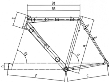
D2 CICLOCROSS ZURIGO Alu
