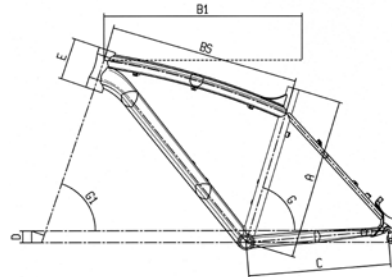
MTB - JAB Alu
