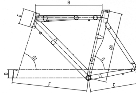
D2 CRONO-TRIATHLON Alu
