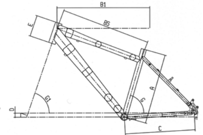
MTB - BIKEMOTARD Alu DUEL Man 26" Alu
